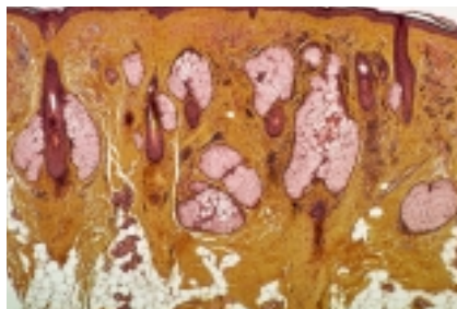
Pelle della fronte
