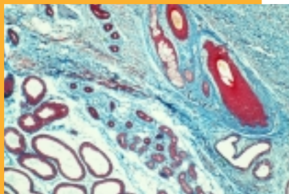
Pelle della regione ascellare
